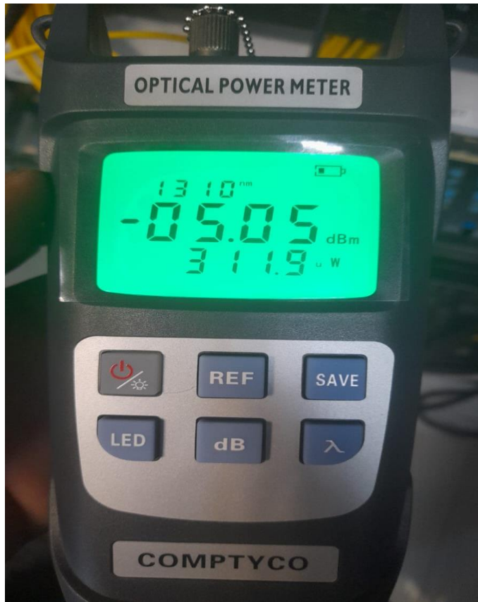
Figura 34. Medida de transmisión del equipo Datacom
