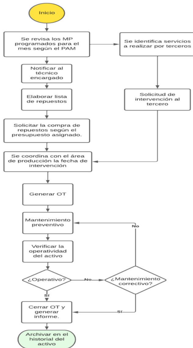
42 Figura 52. Flujograma de mantenimiento preventivo
