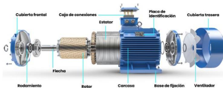
Figura 12. Partes generales de un motor trifásico
