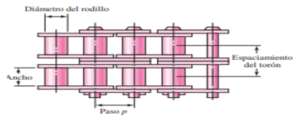
Figura 13. Estructura de transmisión por cadena
