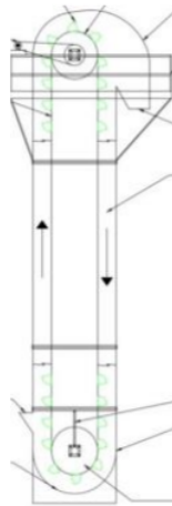
Figura 17. Esquema de un elevador de cangilones
