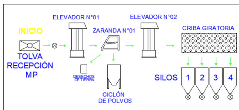
Figura 18. Plano de flujo de procesos – Proceso de pre limpieza
