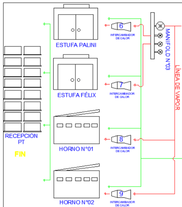
Figura 23. Plano de flujo de procesos – Proceso de secado
