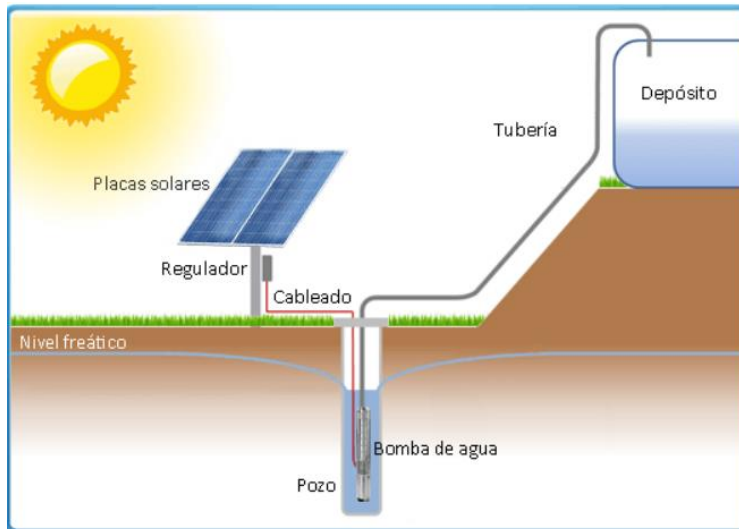
Sistema de bombeo solar directa
