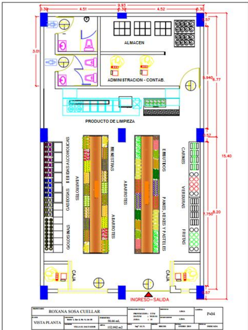
Imagen N° 60 Plano de Distribución de Área de Trabajo
